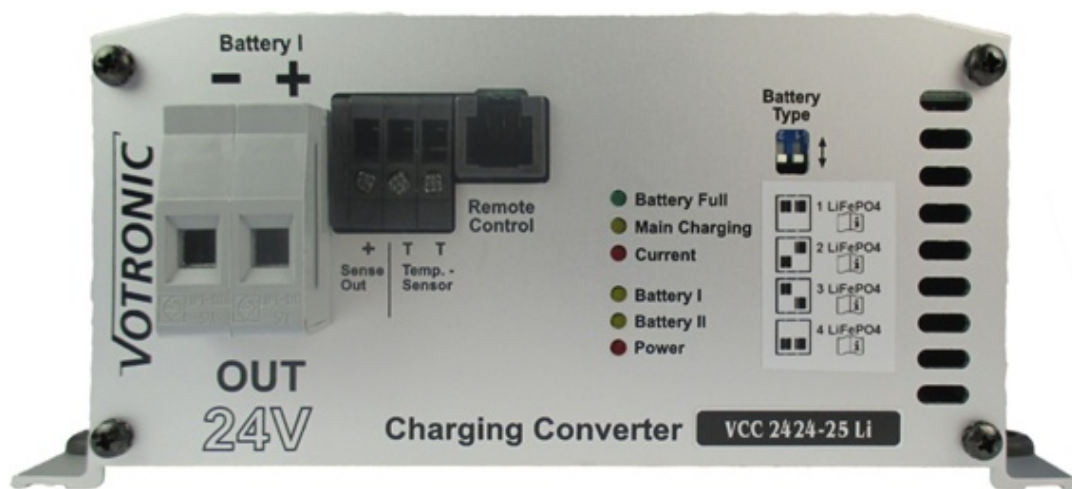
Ansicht Frontplatte Ausgang
